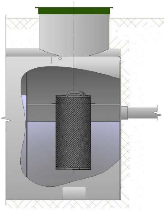
Рис. 1. Фильтрующий патрон в составе: а – ливневого колодца, б – в составе канализационного септика
