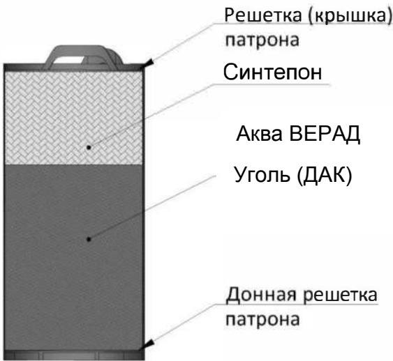
Рис. 3. Загрузка патрона фильтрующим
