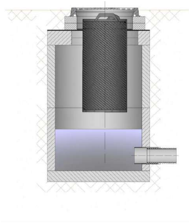
Рис. 1. Фильтрующий патрон в составе: а – ливневого колодца, б – в составе канализационного септика
